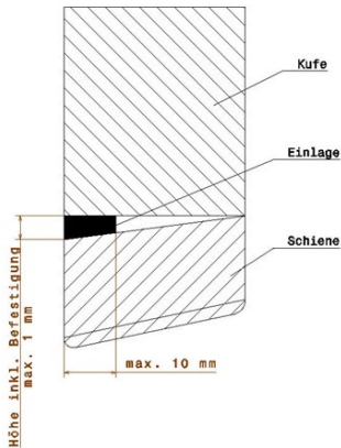
Schnitt A-A:
